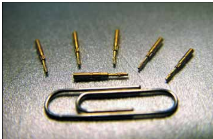
Рис. 10. Контакты Twist pin
