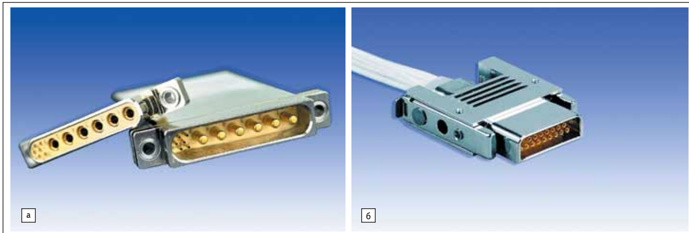
Рис. 3. Разъемы Micro-D: а) с комбинированными контактами; б) Micro-D с защелками
